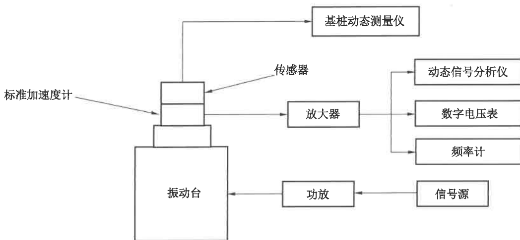
图 1 检定原理示意图
