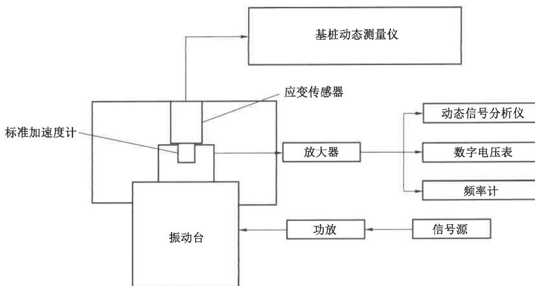
图4 应变测量系统检定框图
