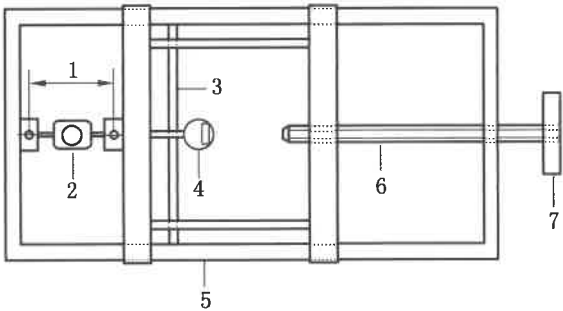
图 3 应变测量装置
