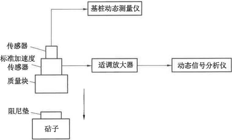
图 2 检定原理图
